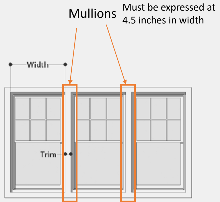
Grouped Window
