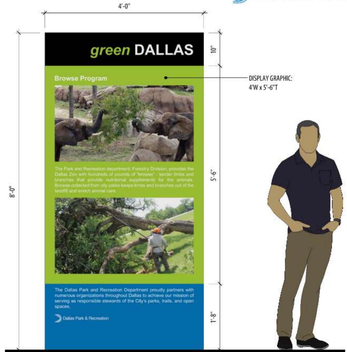
KIOSK ELEVATION
